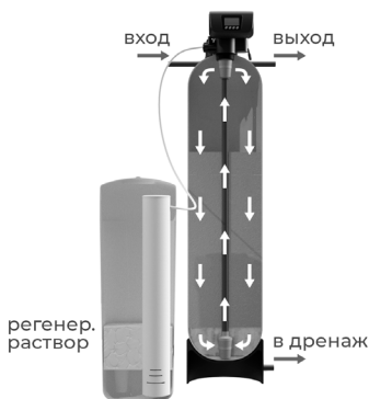
1. Обратная промывка
